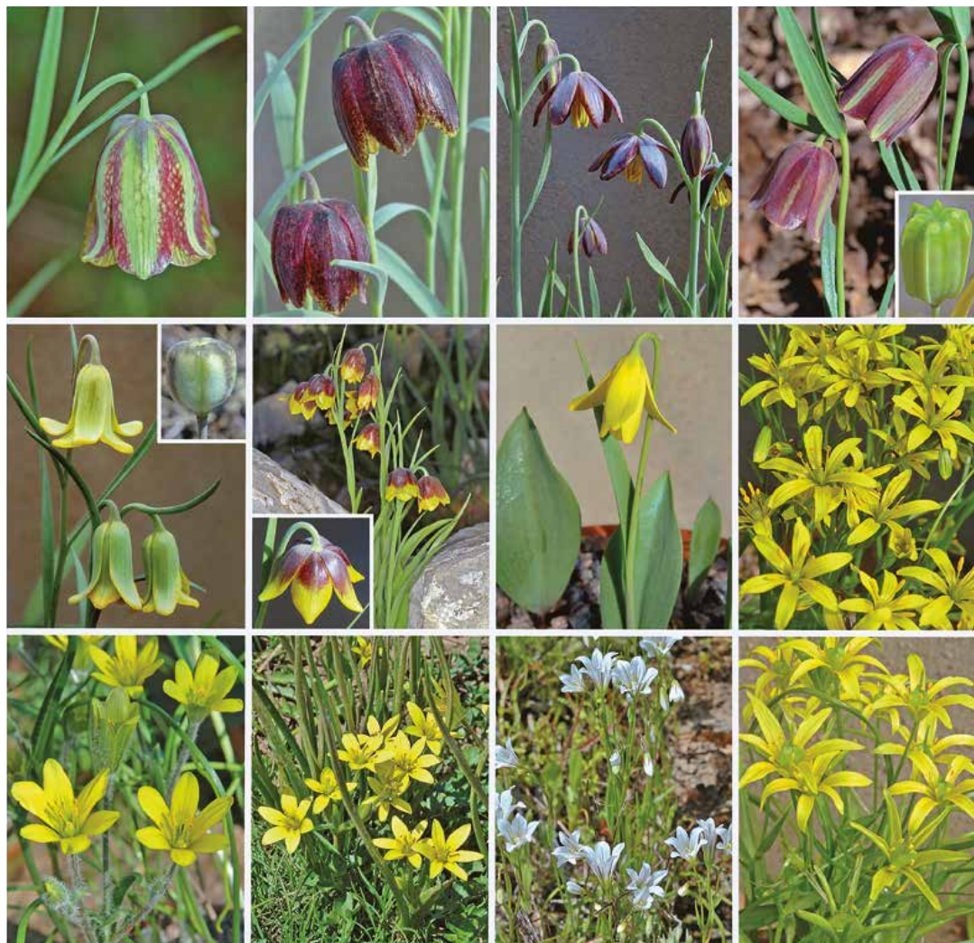
1. Liliaceae: Fritillaria messanensis subsp. messanensis (Olimbos). - 2. Fritillaria montana (Florinis, Mt Boutsis). - 3. Fritillaria obliqua subsp. tuntasiana (Kithnos). - 4. Fritillaria pontica (Athos peninsula). - 5. Fritillaria rhodia (Rodos). - 6. Fritillaria rhodocanakis (Idra). - 7. Fritillaria sibthorpiana (Turkey, Muğla, E of Bozburu). - 8. Gagea amblyopetala (Achaïas, E of Pírgaki). - 9. Gagea dubia (Argolidos, Mt Didimo). - 10. Gagea fragifera (Falakron). - 11. Gagea graeca (Naxos). - 12. Gagea heldreichii (Kriti, Irakliou, Kofinas Oros).
